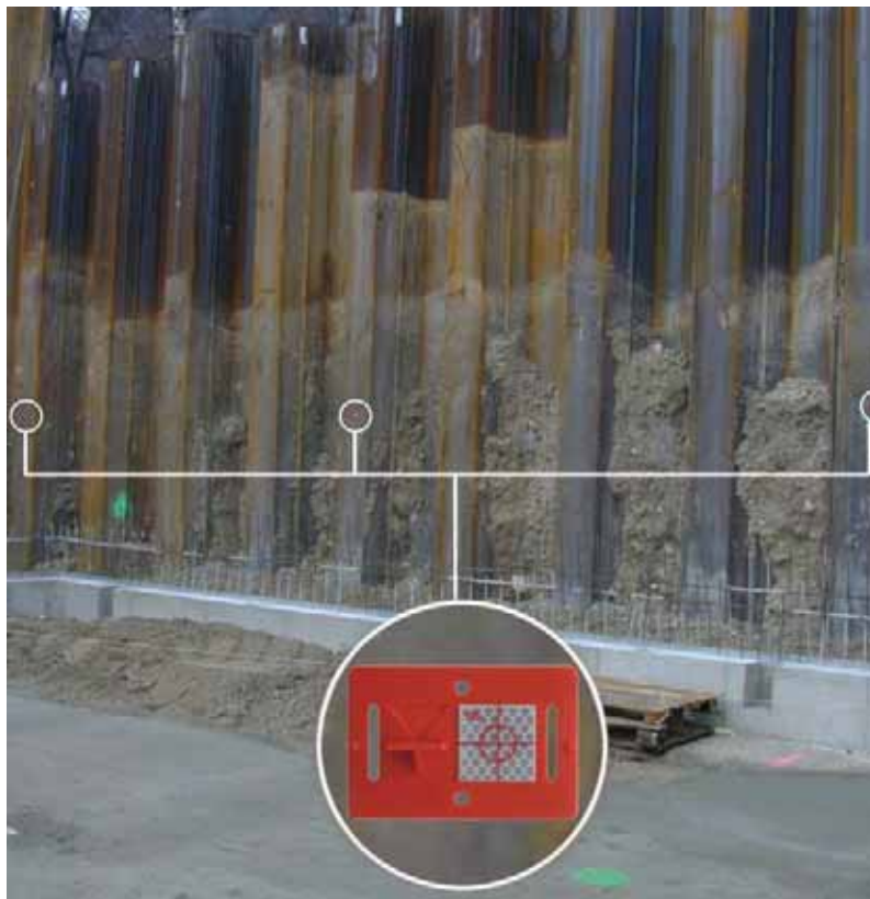
Osservazione di palancolate con RS30r
